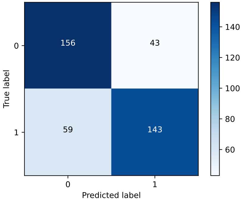
Confusion Matrix - PCA_SVM (last fold)
