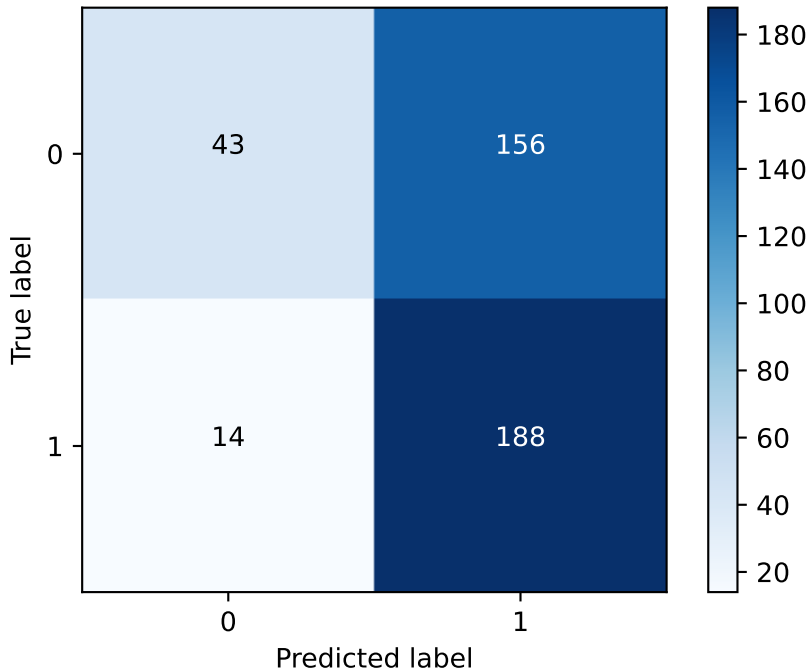
Confusion Matrix - BAYES_OPT_SVMS (last fold)
