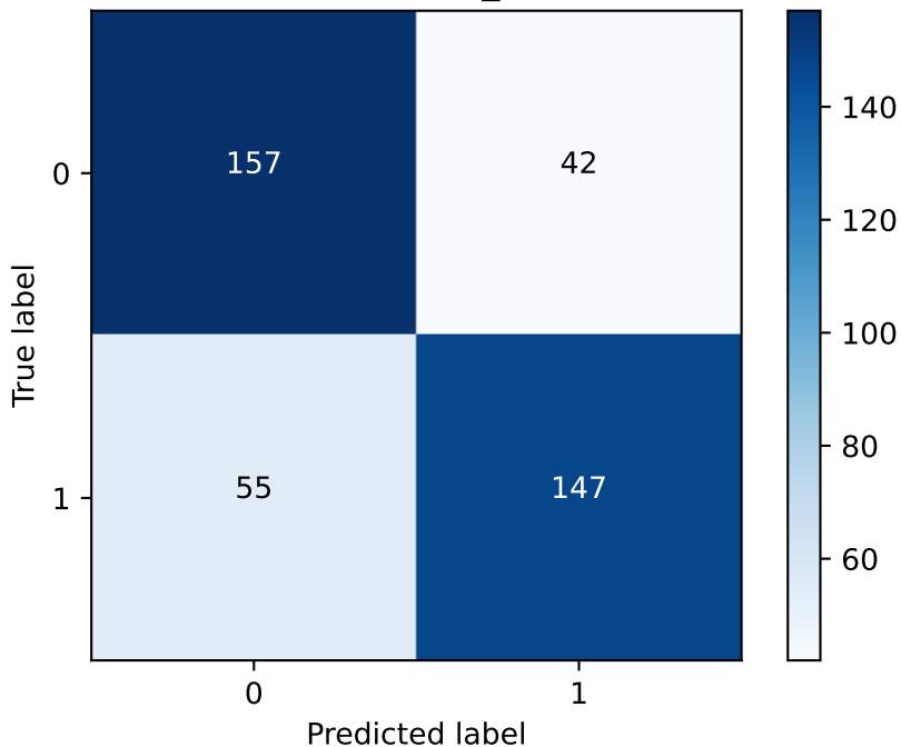
Confusion Matrix - PSO_SVM (last fold)
